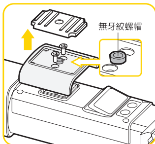
更換電子秤上蓋
